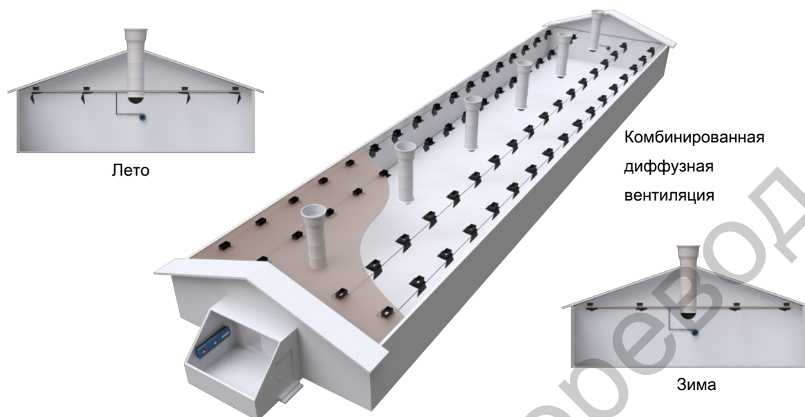
Рисунок 8: Комбидиффузная система объединяет лучшие характеристики двух систем вентиляции: диффузную систему и систему с низким потреблением энергии.
