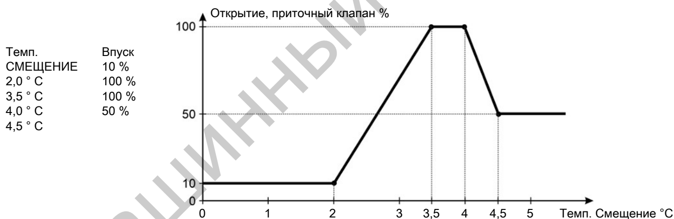
Рисунок 10: Комбидиффузный приточный клапан – уменьшение бесступенчатого открытия при высокой внешней температуре
