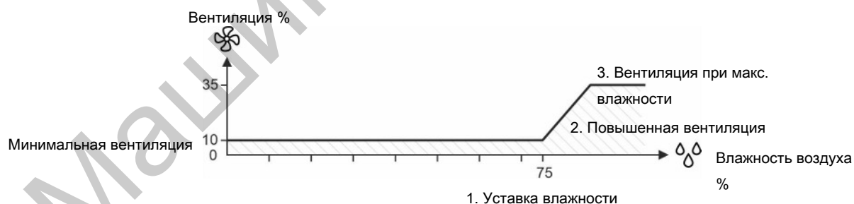
Рисунок 14: Вентиляция с увлажнением: 1. Влажность воздуха превышает уставку увлажнения 2. Контроллер увеличивает вентиляцию. 3. Увеличьте вентиляцию до максимальной влажности (35%).
