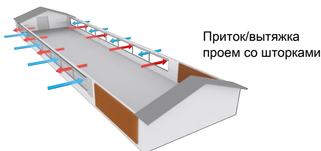
Рисунок 20: Пример помещения с естественной вентиляцией, применяемой вместе с туннельной вентиляцией, естественная вентиляция.
