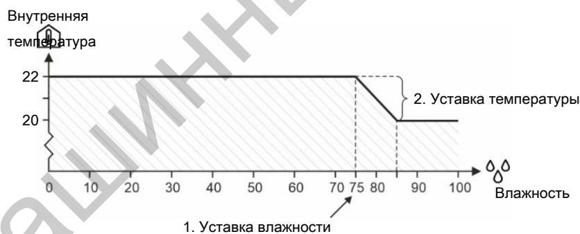
Рисунок 15: Управление влажностью со снижением температуры
