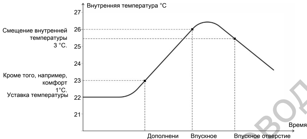
Рисунок 9: Комбидиффузный приточный клапан – регулировка внутренней температуры
