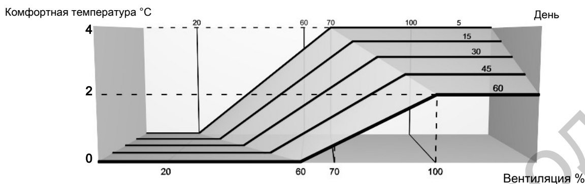
Рисунок 5: Комфортная температура при производстве партии
