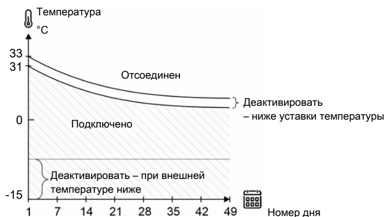
Рисунок 18: Рекуператор тепла – нижний и верхний пределы внешней температуры
